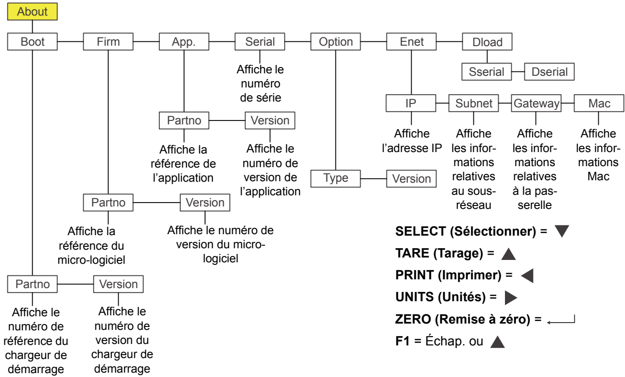
Figure 4.3 Menu About (À propos)
