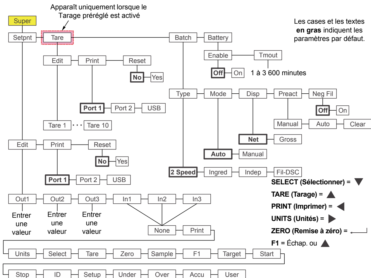
Figure 7.5 Menu Supervisor (Superviseur) pour l'application Mise en lots
