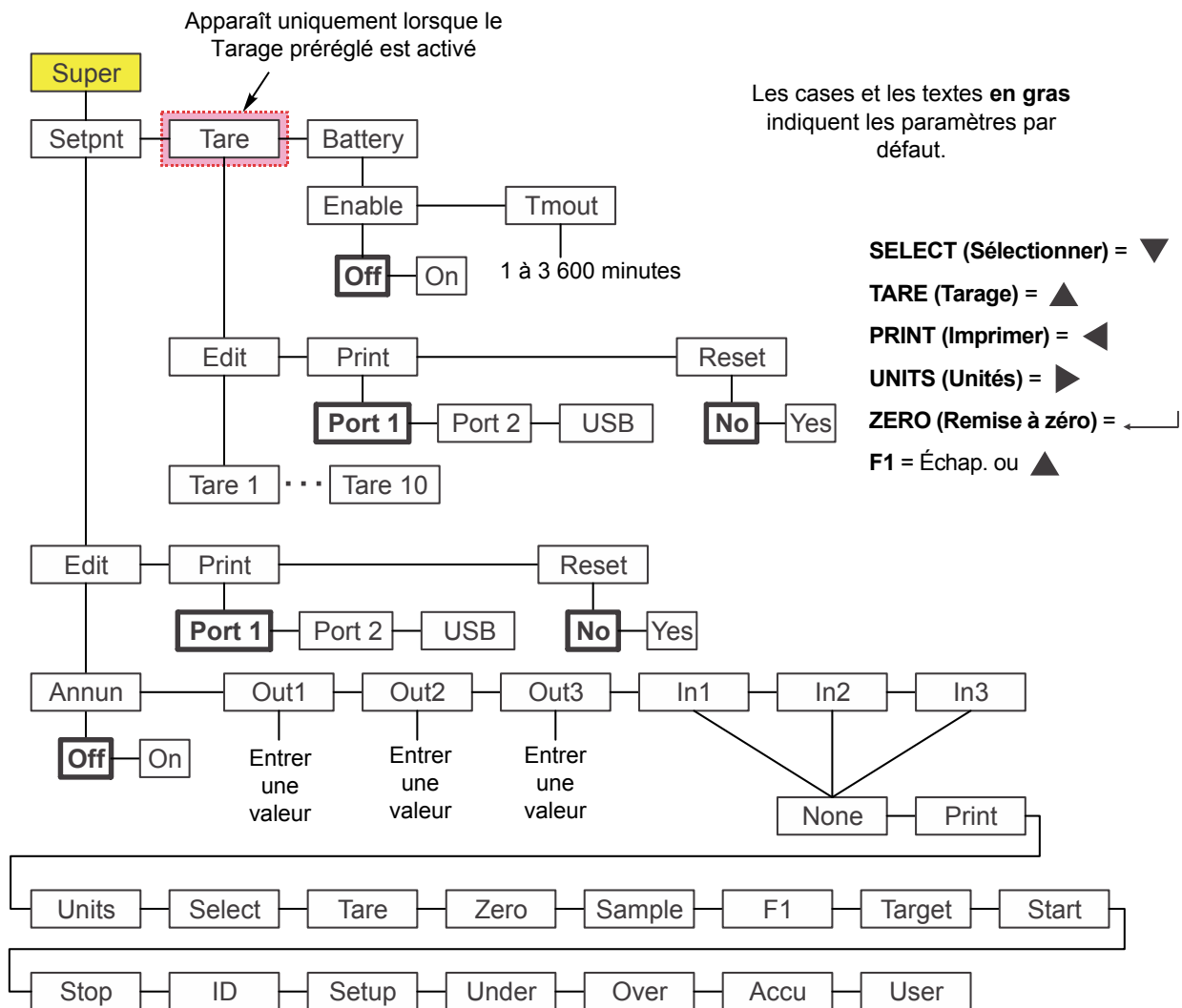
Figure 7.1 Menu Supervisor (Superviseur) pour l'application Pesée générale
