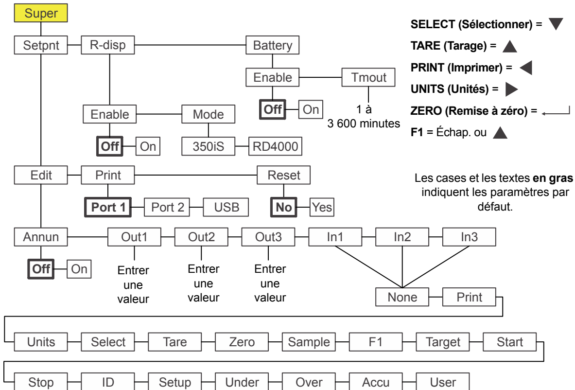
Figure 7.7 Menu Supervisor (Superviseur) de l'application Affichage à distance
