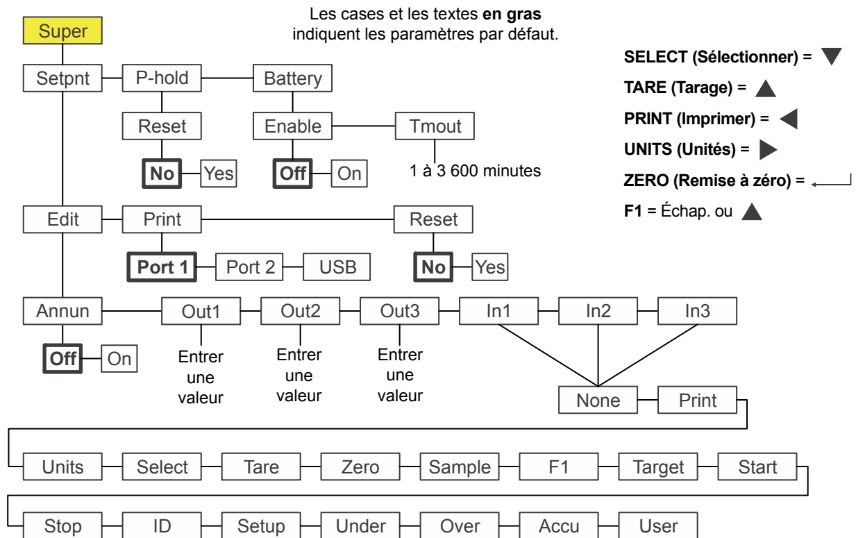
Figure 7.6 Menu Supervisor (Superviseur) de l'application Retenue de crête
