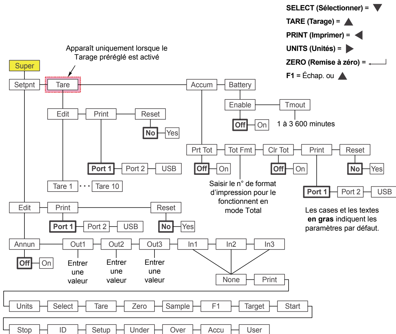
Figure 7.2 Menu Supervisor (Superviseur) pour l'application Accumulateur
