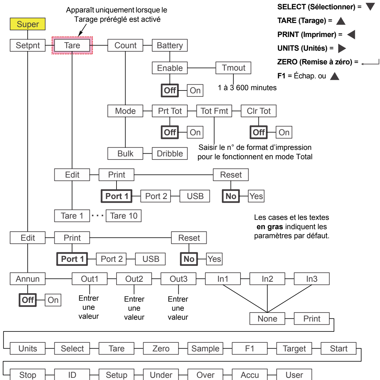
Figure 7.3 Menu Supervisor (Superviseur) pour l'application Comptage
