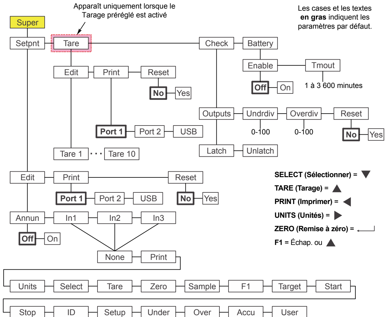
Figure 7.4 Menu Supervisor (Superviseur) pour l'application Contrôle de poids
